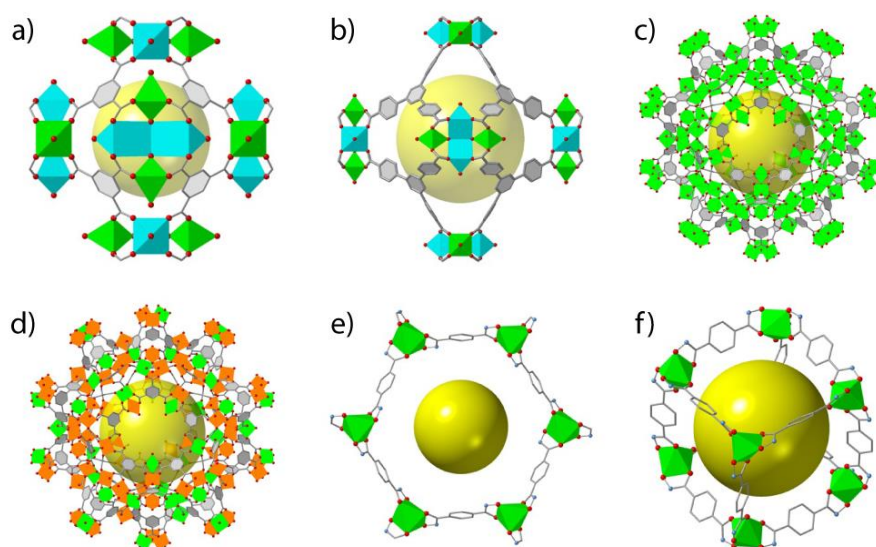
Structure of homo- and heterometallic Ti-MOFs: a) MUV-10, b) MUV-12, c) MIL-100(Ti), d) MUV-101(M), e) MUV-11 and f) cMUV-11. MUV stands for Materials of the Universidad de València.
