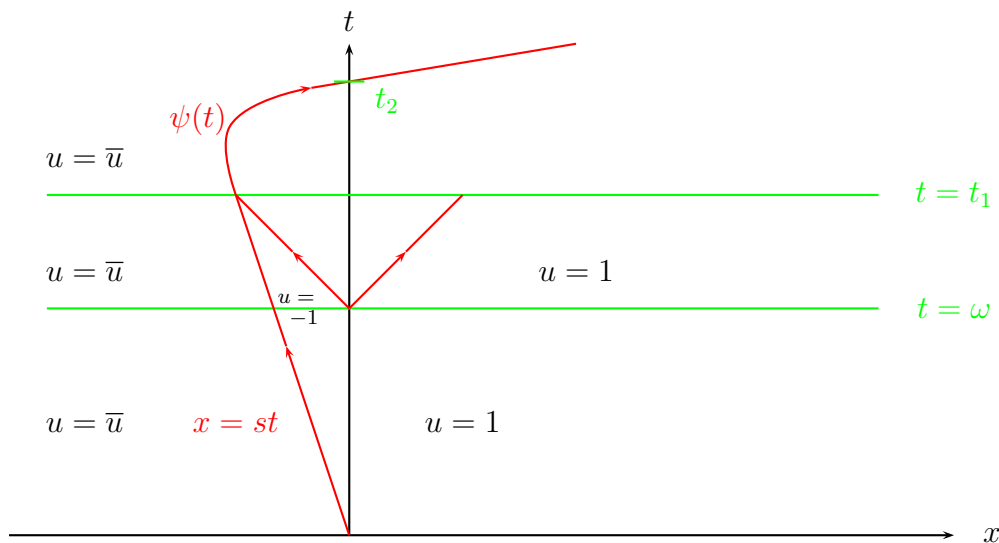
Abbildung 1.4: Schockkurve für \bar{u} > 0
