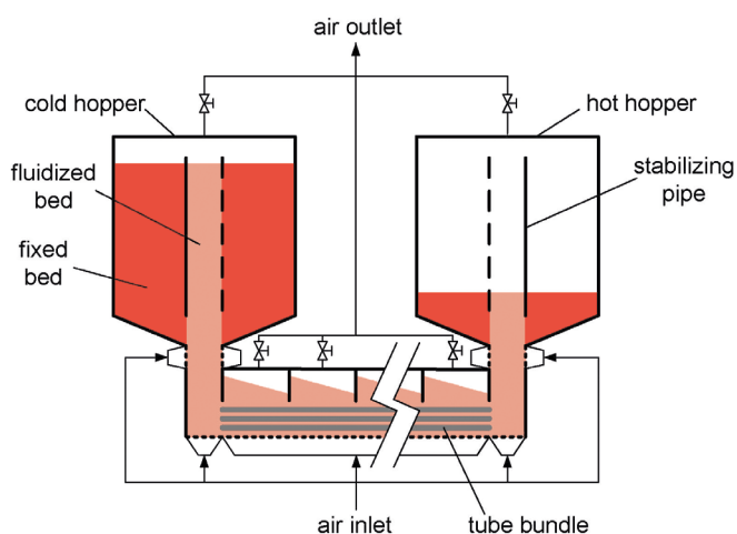
Prinzipskizze des FP-TES Wärmespeichers
