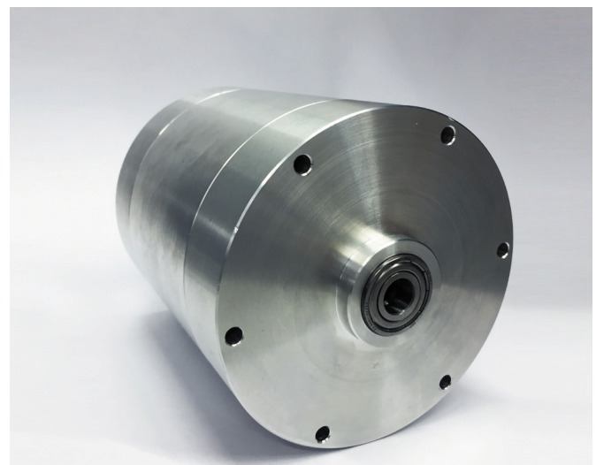
Sensorlos geregelter Synchronmotor ohne Seltenerdmetalle
