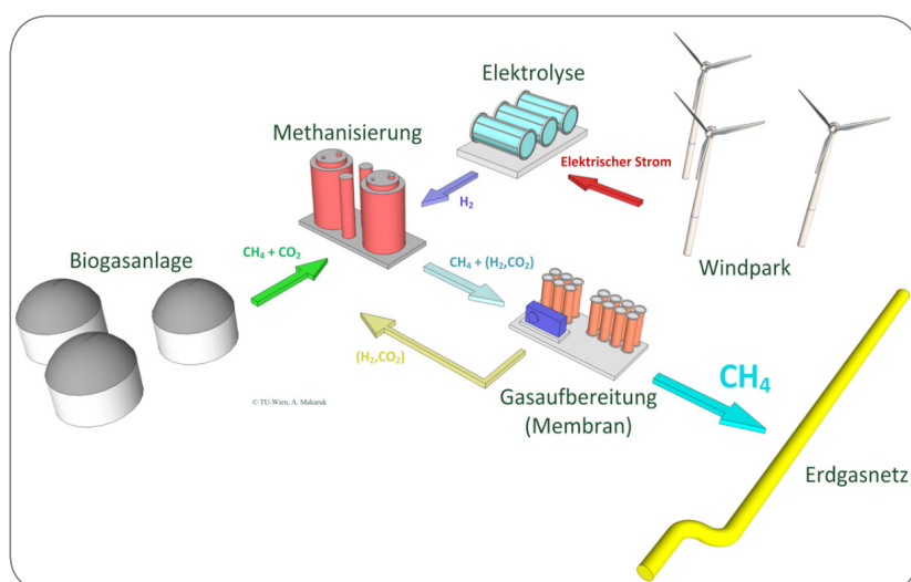
Fließbild des an der TU Wien entwickelten Power-to-Gas Systems
